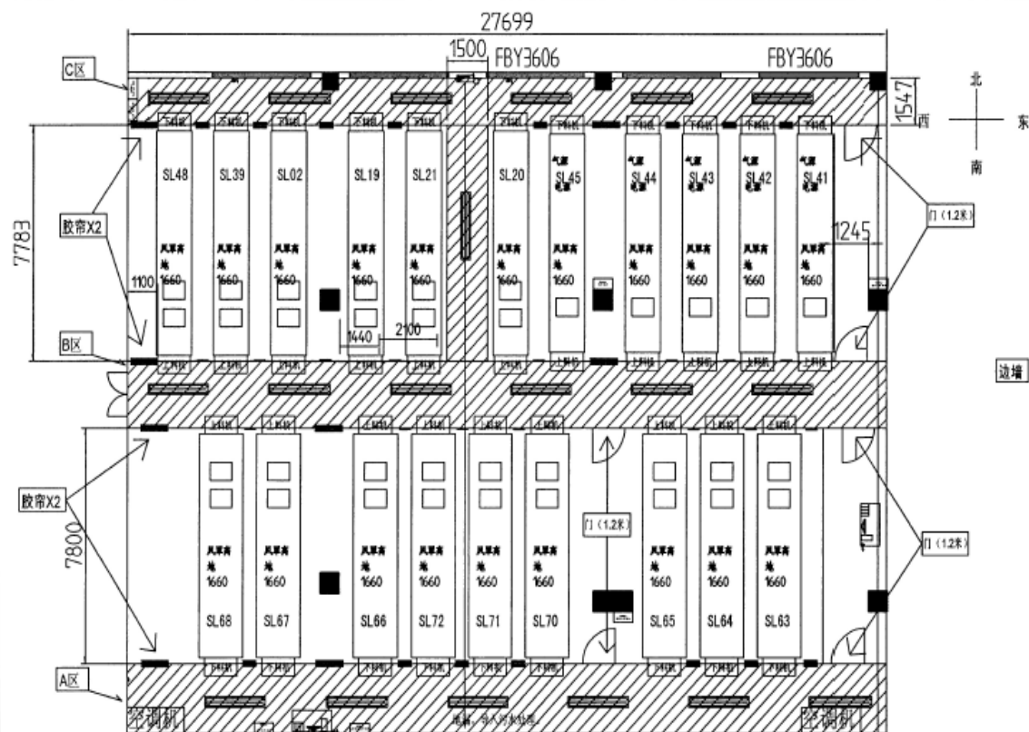
端华新厂房五层烧炉围蔽布局图
